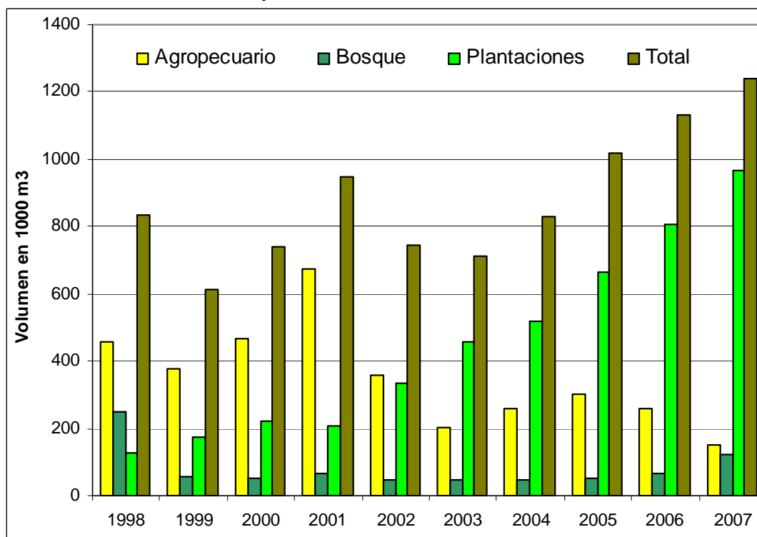
Figura 3 Volumen de madera cosechado por fuente en Costa Rica 1998-2007.
